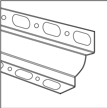
PROFILO profile · Leiste · profil · perfil · профиль · 外形
