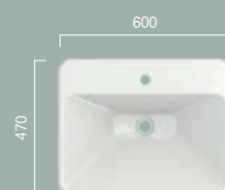
LW170YBT1#XW Möbelwaschtisch 600 mm mit Hahnloch, ohne Überlauf Furniture washbasin 600 mm with tap hole, without overflow
